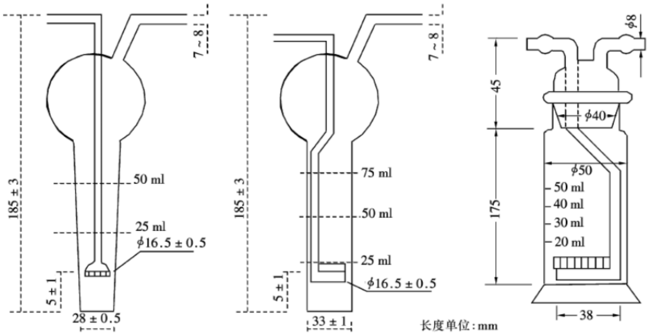
图 4-2 多孔玻璃吸收瓶（管）结构示意图
