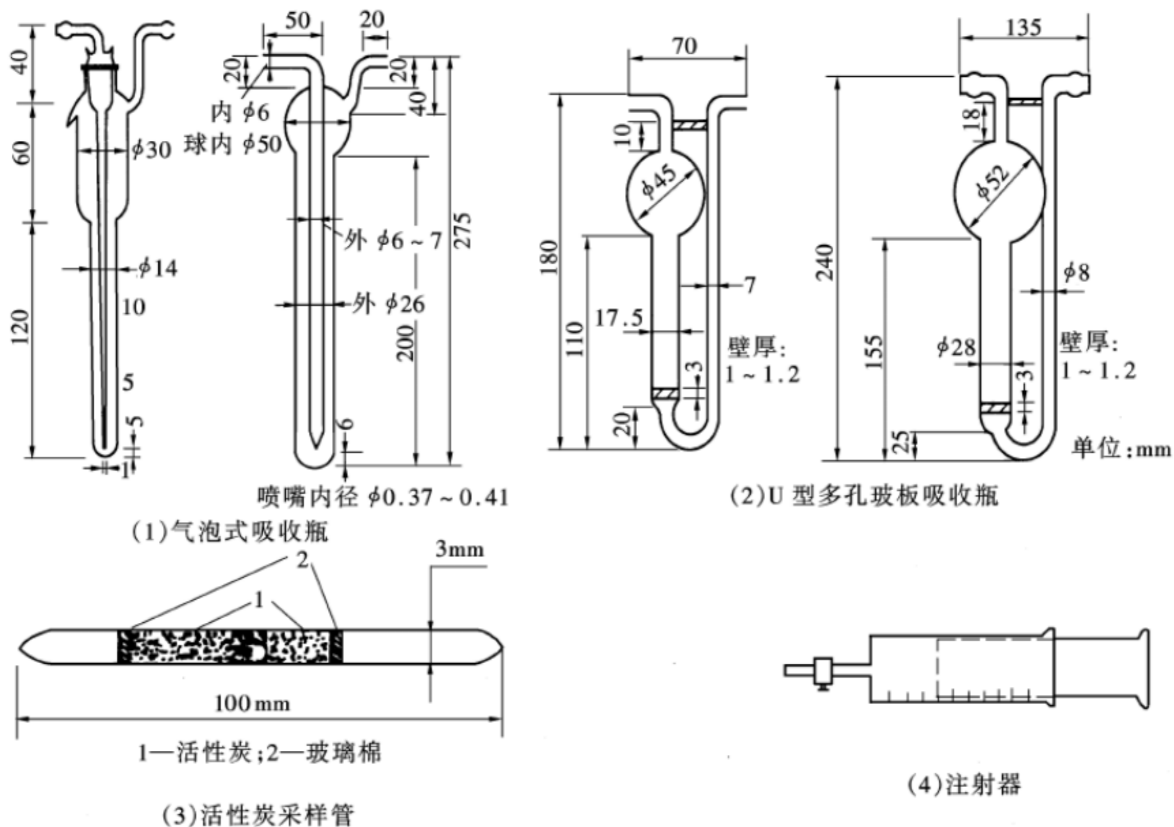
图 4-5 部分气样捕集装置结构示意图
