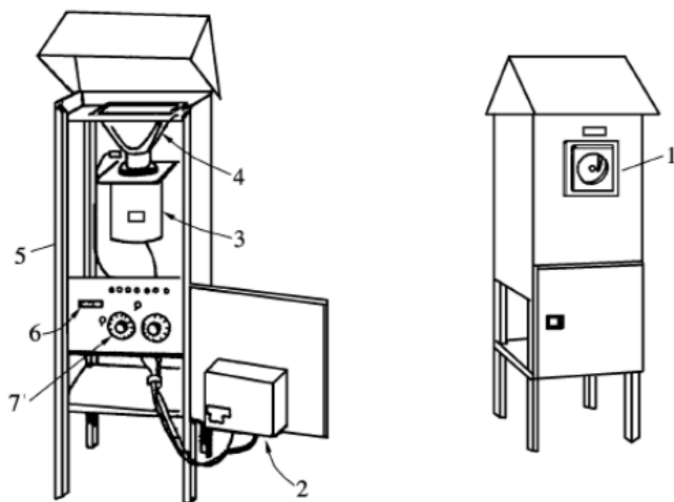
1—流量记录器；2—流量控制器；3—抽气风机；4—滤膜夹； 5—铝壳；6—工作计时器；7—计时器的程序控制器
