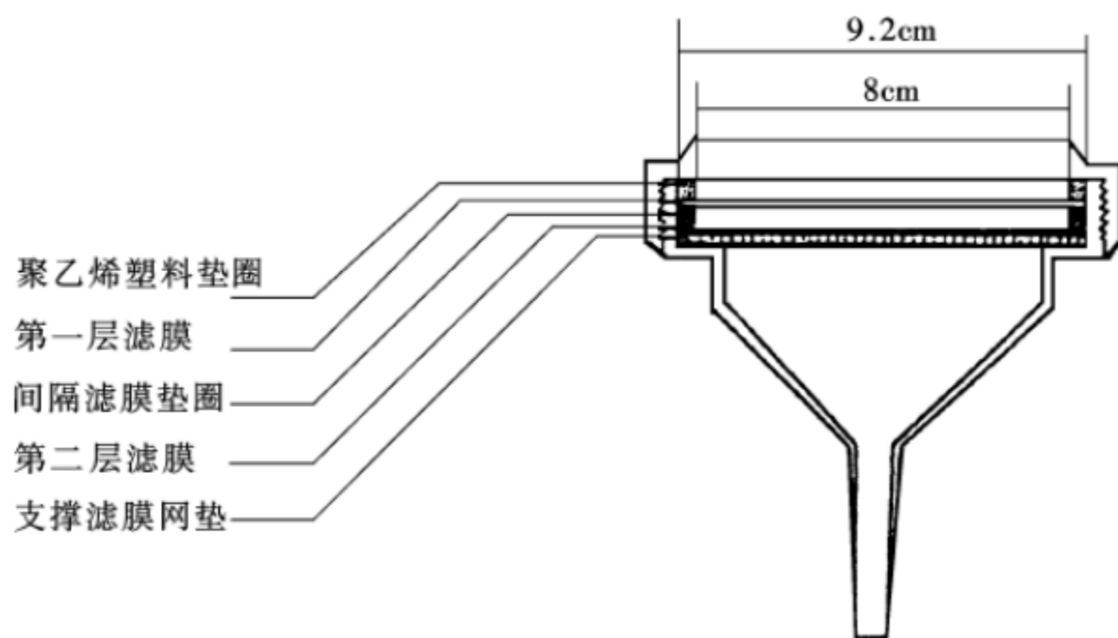
(2) 中流量采样头结构示意图
