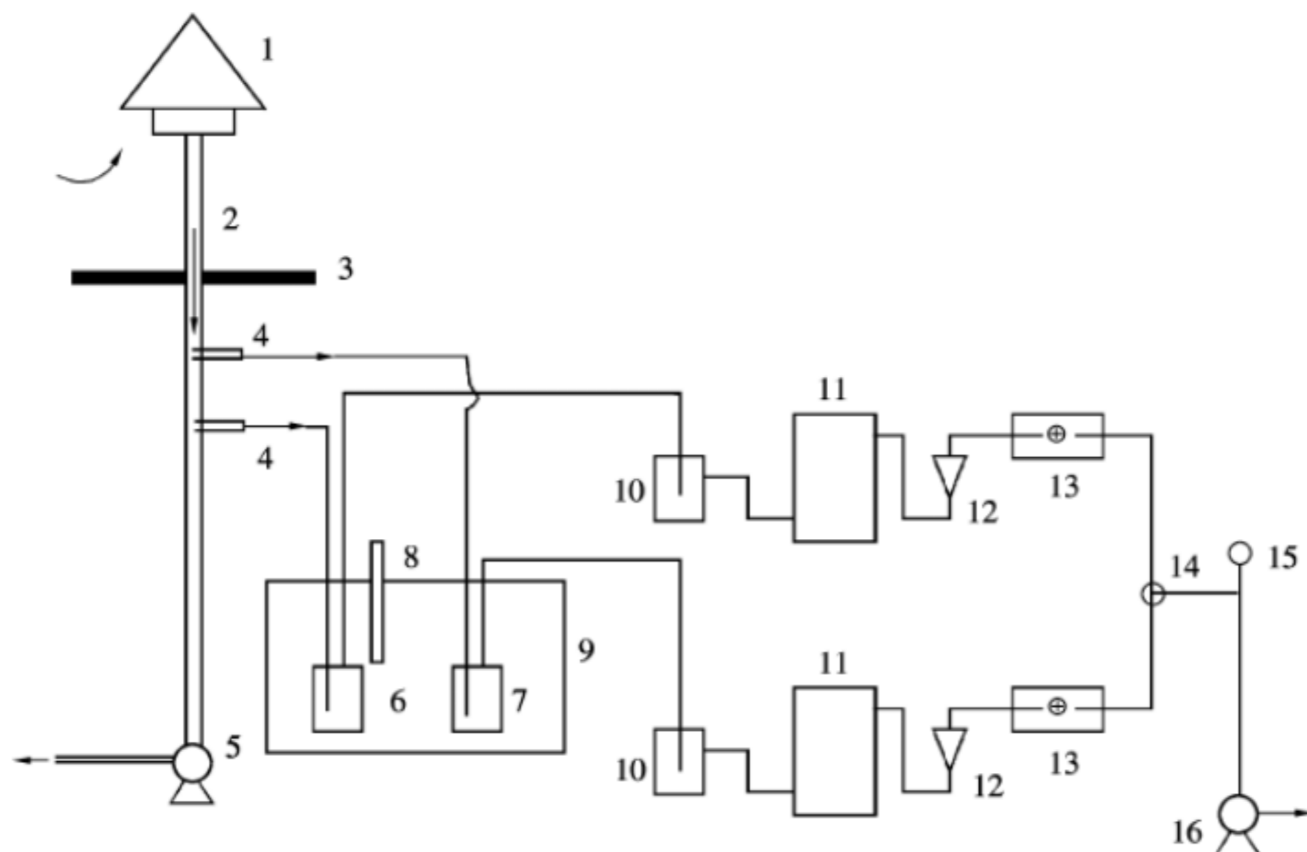
1—采样头；2—采样总管；3—采样亭屋顶；4—采样支管；5—引风机；6—二氧化氮吸收瓶；7—二氧化硫吸收瓶；8—温度计；9—恒温装置；10—滤水井；11—干燥器；12—转子流量计；13—限流孔；14—三通阀；15—真空表；16—抽气泵
